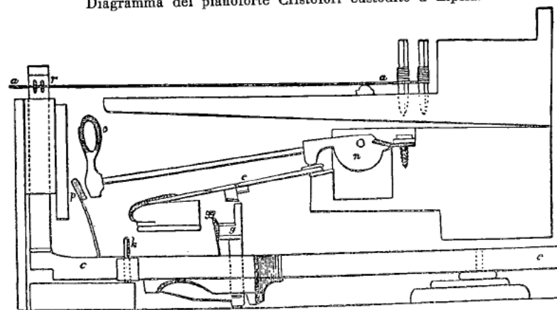
Diagramma del pianoforte Cristofori custodito a Lipsia.
