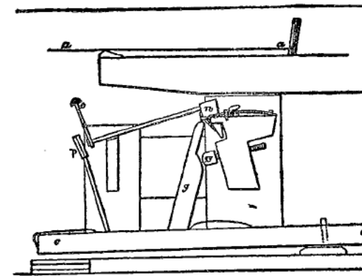
Diagrammi della meccanica di Broadwood (1777-1780)
