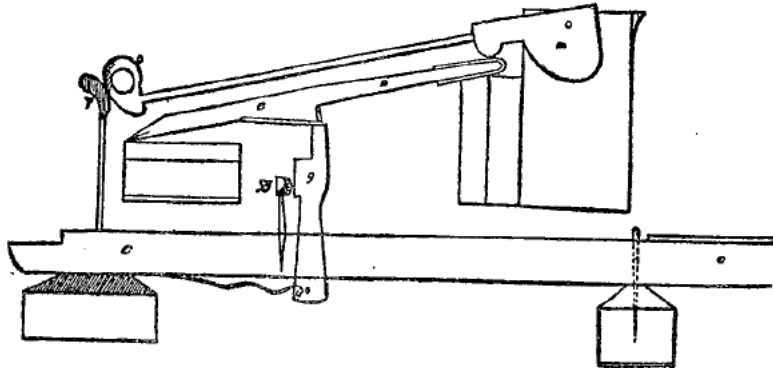
Diagramma della meccanica di Silbermann.
