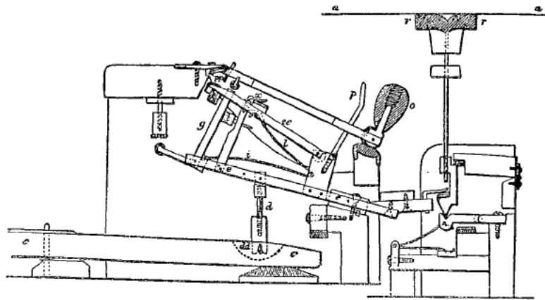
Diagramma della meccanica di Erard.
