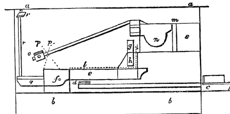
Diagramma della meccanica del pianoforte Cristofori, custodito nel Metropolitan Museum di Nuova York. (v. Tav. V)
